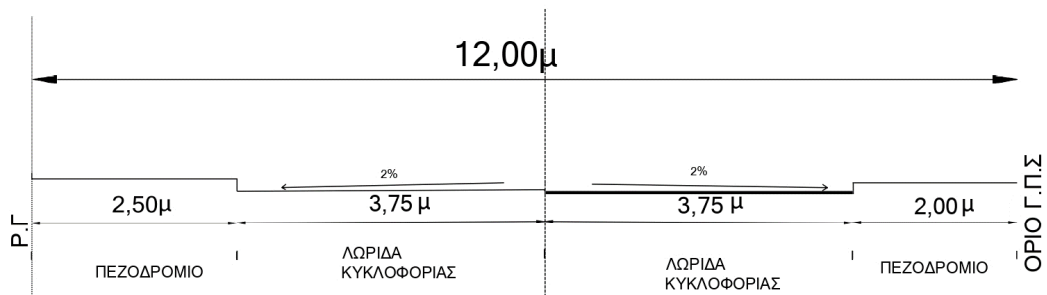
Εικ.2 Τυπική διατομή οδού Αισώπου
