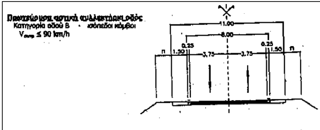
Εικ. 1. Συνήθης διατομή πρωτεύουσας αστικής συλλεκτήριας οδού 1
