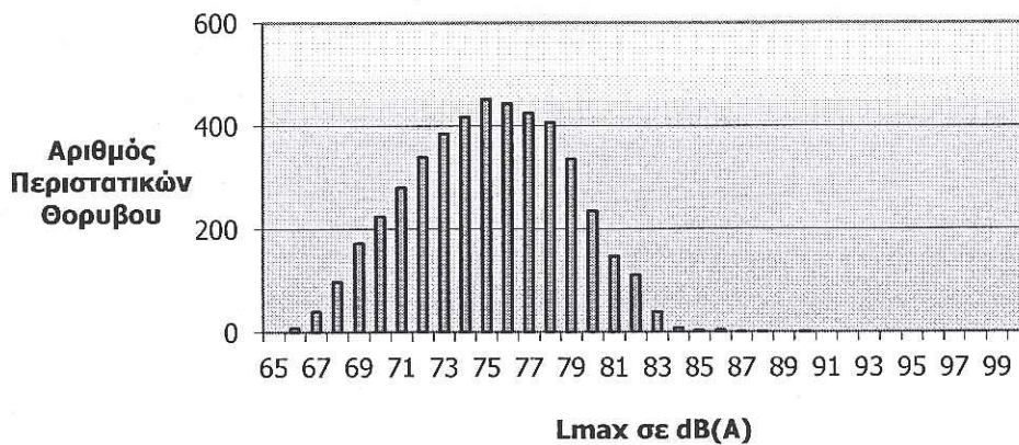
Κατανομή Στάθμης Θορύβου L_{max} Σταθμός: Αγ. Ιωάννης (NMT 3) Συνολικός Αριθμός Συσχετισμένων Περιστατικών Θορύβου: 4578
