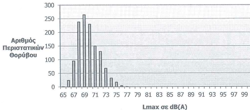
Κατανομή Στάθμης Θορύβου L_{max} Σταθμός: Αρτέμιδα (NMT 5) Συνολικός Αριθμός Συσχετισμένων Περιστατικών Θορύβου: 1254
