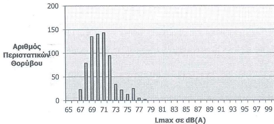
Κατανομή Στάθμης Θορύβου L_{max} Σταθμός: Αγία Κυριακή (NMT 4) Συνολικός Αριθμός Συσχετισμένων Περιστατικών Θορύβου: 716
