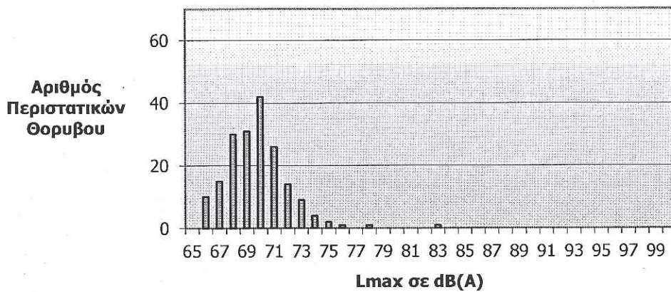
Κατανομή Στάθμης Θορύβου L_{max} Σταθμός: Βορινέζα (NMT 2) Συνολικός Αριθμός Συσχετισμένων Περιστατικών Θορύβου: 186
