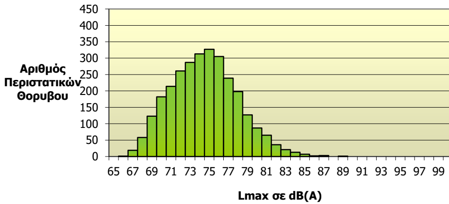
Κατανομή Στάθμης Θορύβου L_{max} Σταθμός: Αγ. Ιωάννης (NMT 3) Συνολικός Αριθμός Συσχετισμένων Περιστατικών Θορύβου: 2889
