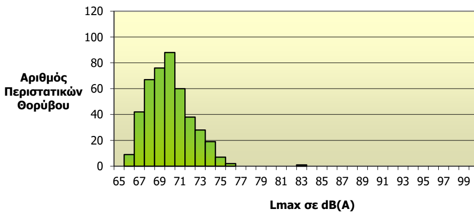
Κατανομή Στάθμης Θορύβου L_{max} Σταθμός: Αρτέμιδα (NMT 5) Συνολικός Αριθμός Συσχετισμένων Περιστατικών Θορύβου: 437
