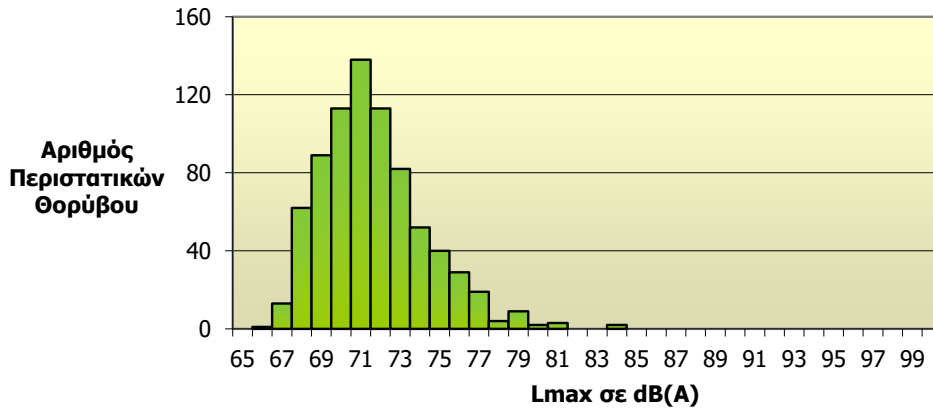
Κατανομή Στάθμης Θορύβου L_{max} Σταθμός: Αγία Κυριακή (NMT 4) Συνολικός Αριθμός Συσχετισμένων Περιστατικών Θορύβου: 771
