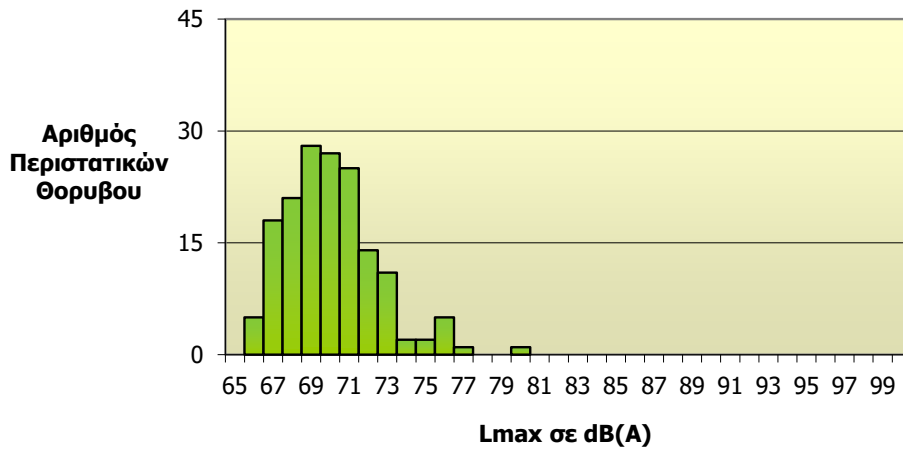
Κατανομή Στάθμης Θορύβου L_{max} Σταθμός: Βορινέζα (NMT 2) Συνολικός Αριθμός Συσχετισμένων Περιστατικών Θορύβου: 160
