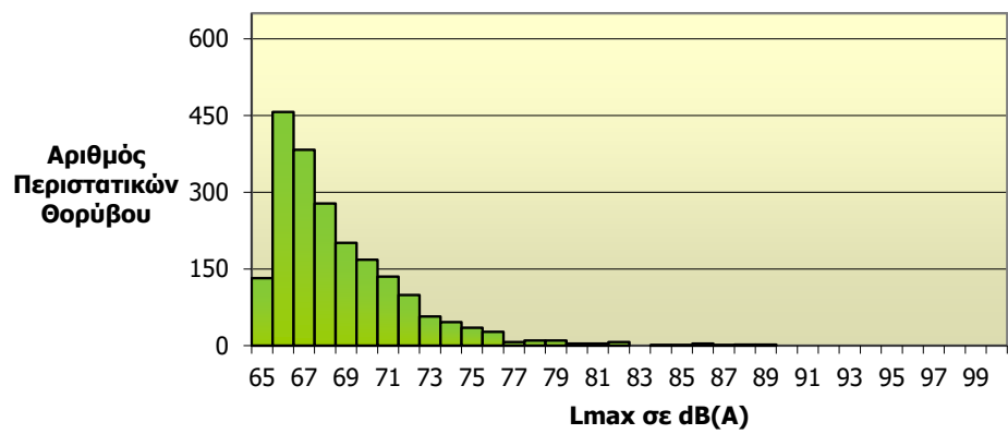
Κατανομή Στάθμης Θορύβου L max Σταθμός: Αγία Κυριακή (NMT 4) Συνολικός Αριθμός Συσχετισμένων Περιστατικών Θορύβου: 2071
