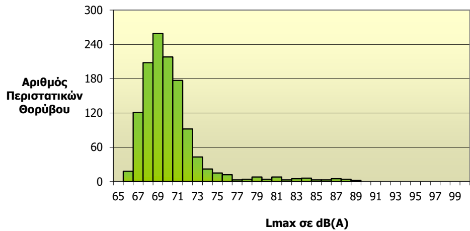
Κατανομή Στάθμης Θορύβου L max Σταθμός: Αρτέμιδα (NMT 5) Συνολικός Αριθμός Συσχετισμένων Περιστατικών Θορύβου: 1243
