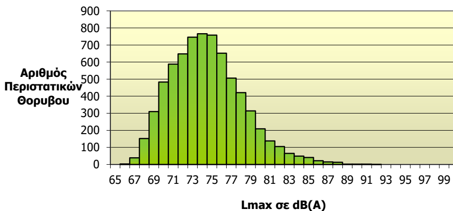
Κατανομή Στάθμης Θορύβου L_{max} Σταθμός: Αγ. Ιωάννης (NMT 3)
