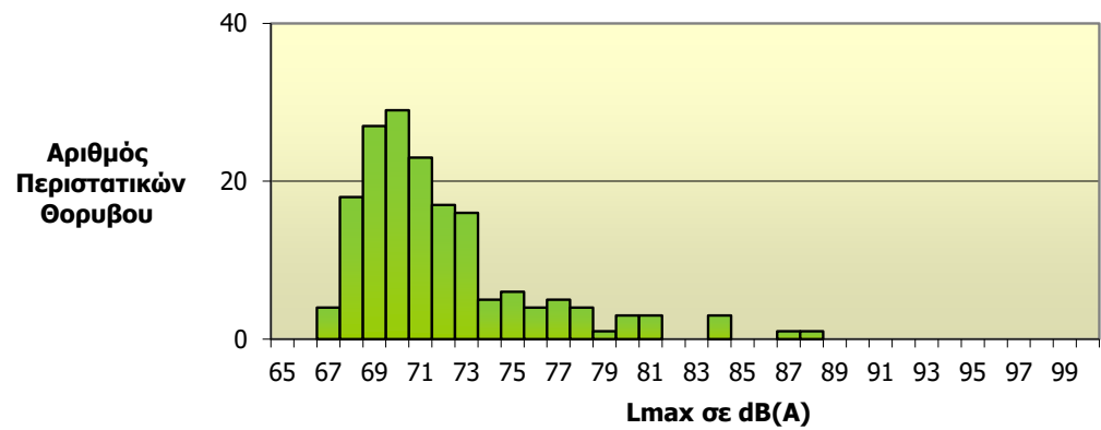
Κατανομή Στάθμης Θορύβου Lmax Σταθμός: Μαρκόπουλο (NMT 8) Συνολικός Αριθμός Συσχετισμένων Περιστατικών Θορύβου: 170
