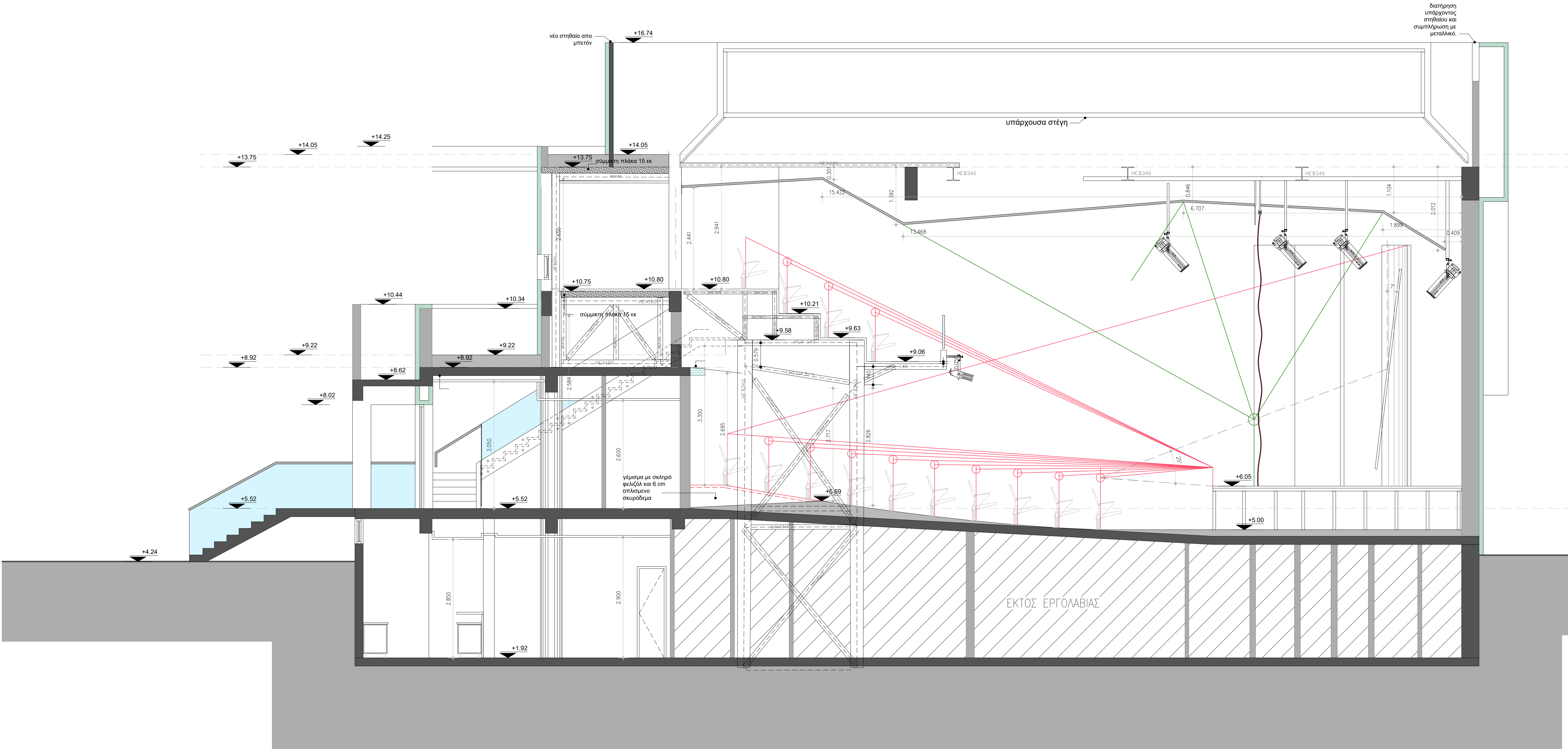
ΤΟΜΗ Α-Α
