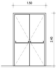
ΔΙΦΥΛΛΗ ΘΥΡΑ - ΟΨΗ ΚΛ. 1/50
