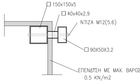
ΛΕΠΤΟΜΕΡΕΙΑ Λ1 ΚΛ 1:10
