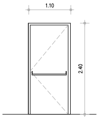
ΜΟΝΟΦΥΛΛΗ ΘΥΡΑ - ΟΨΗ ΚΛ. 1/50
