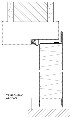
ΠΟΡΤΑ ΠΥΡΑΣΦΑΛΕΙΑΣ ΜΕ ΚΑΣΑ ΧΩΡΙΣ ΣΚΩΤΙΑ ΚΑΘΕΤΗ ΤΟΜΗ
