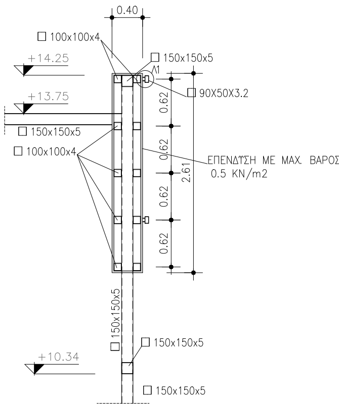
ΤΟΜΗ 1-1 ΚΛ 1:50
