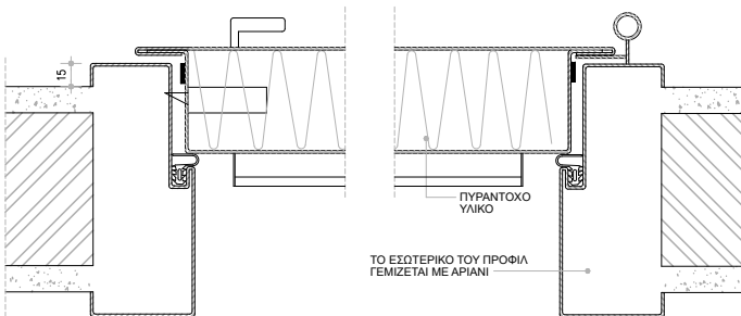
ΟΡΙΖΟΝΤΙΑ ΤΟΜΗ ΜΟΝΟΦΥΛΛΗΣ
